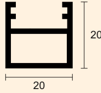
Kalıp No : 1619 Ağırlık : 0,298 kg/m
