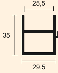
Kalıp No : 1399 Ağırlık : 0,718 kg/m
